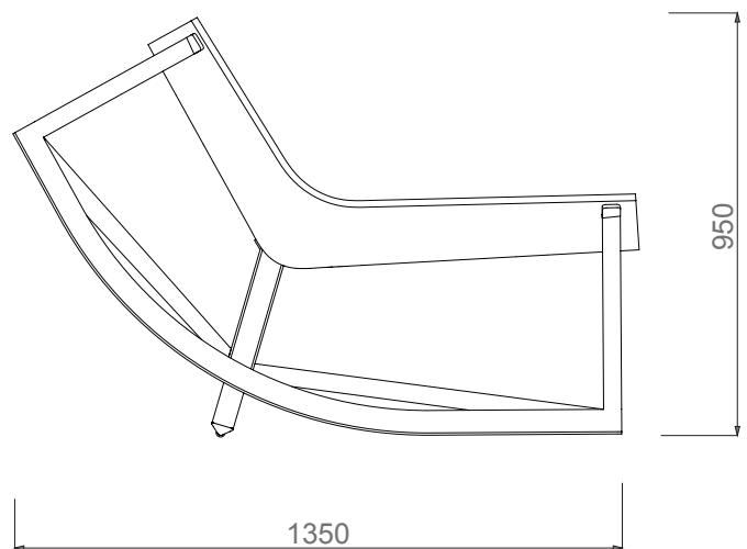
Seitenansicht Position 2 / Side View Position 2
