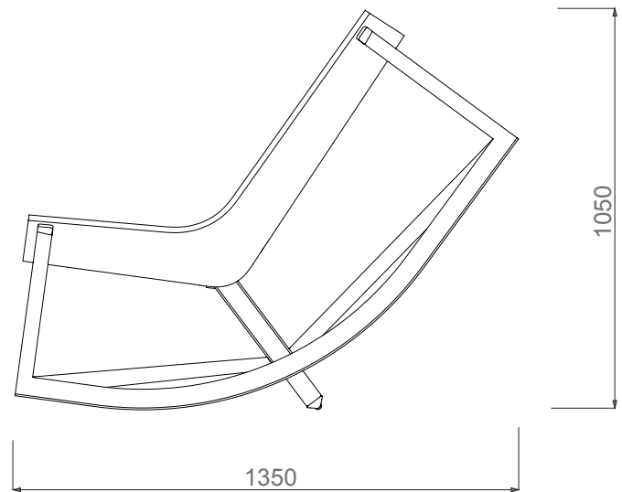
Seitenansicht Position 1 / Side View Position 1
